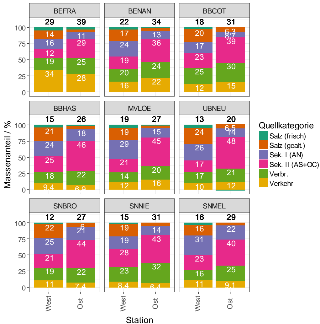
Abbildung 65: Massenananteil der Quellkategorien für die aus der PMF resultierenden PM10- Massekonzentration (schwarze Zahlen über Säulen in \mu\text{g m}^{-3} ) in Abhängigkeit von der Anströmung, dargestellt für alle 9 Messstationen aus Level 1.
